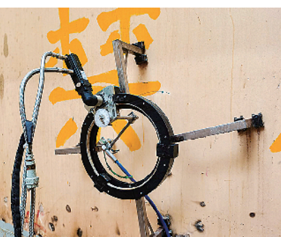
高压水切割设备正在作业
